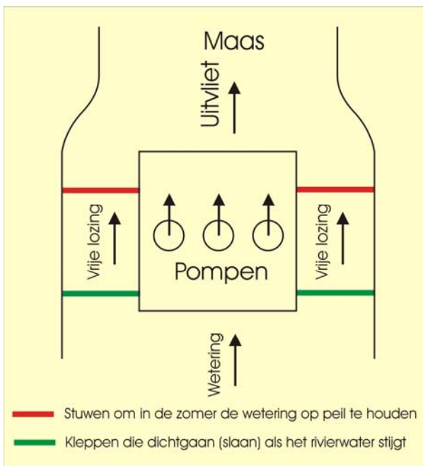
Werking van het gemaal
